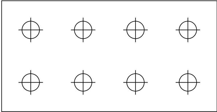
Pile cap 11.1 m x 5.7 m.
